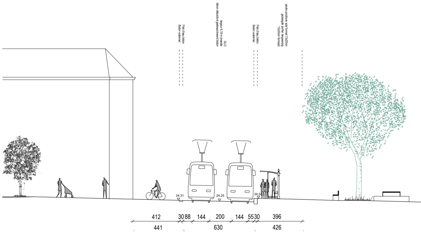
Coupe projeté
