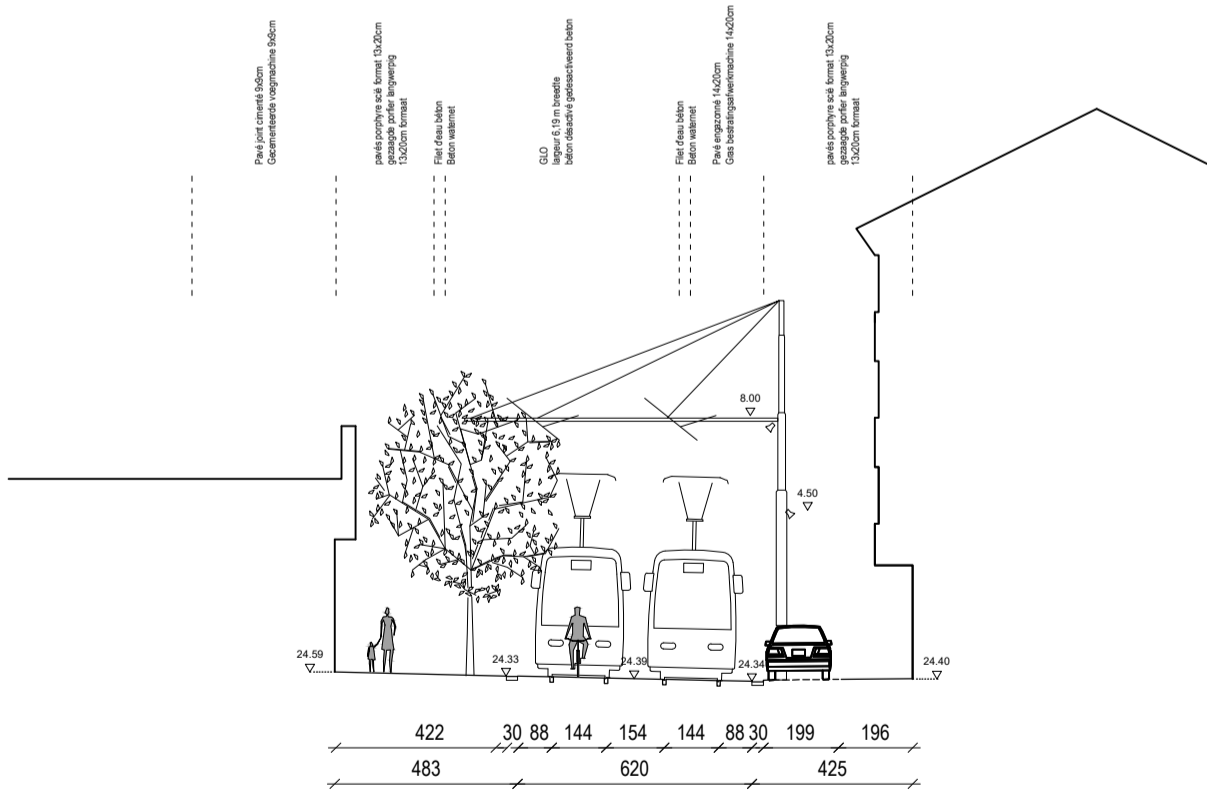
Coupe projeté
